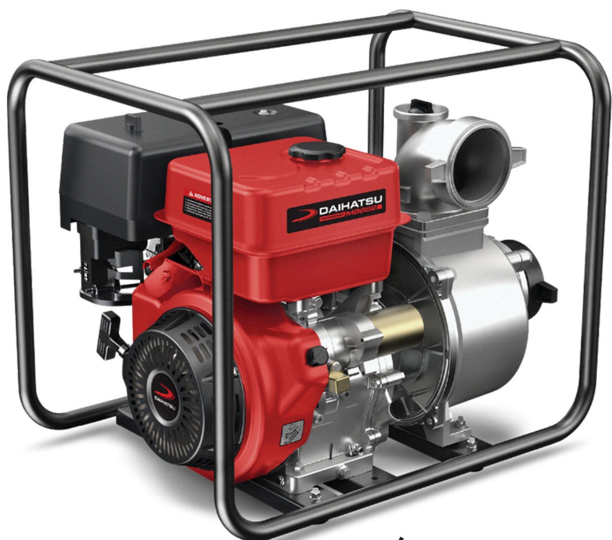
MOTOBOMBA A EXPLOSIÓN - 6,5HP / 196cc / SALIDA DE 2"
