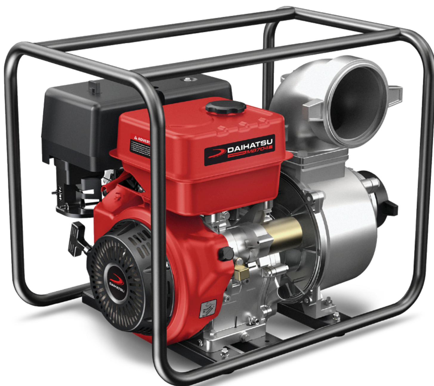
MOTOBOMBA A EXPLOSIÓN - 7,0HP / 208cc / SALIDA DE 4"
